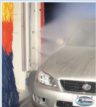
Alta pressione laterale Side High Pressure
